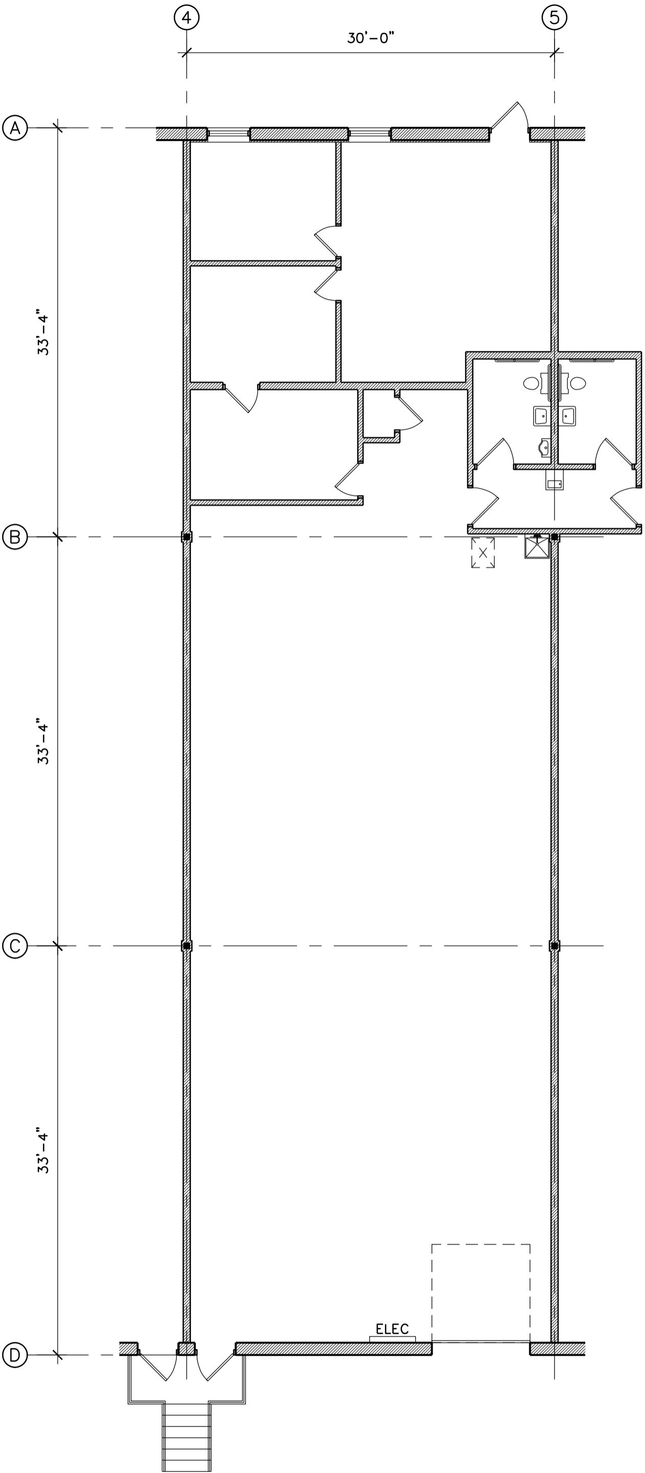
1 FLOOR PLAN LH1 SCALE: 1/8" = 1'-0"
